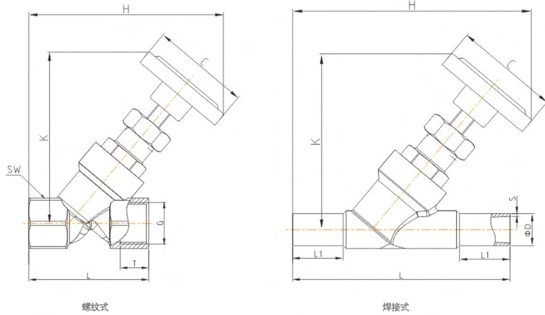
螺纹式
