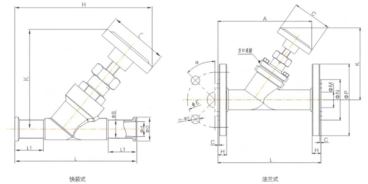
快装式
